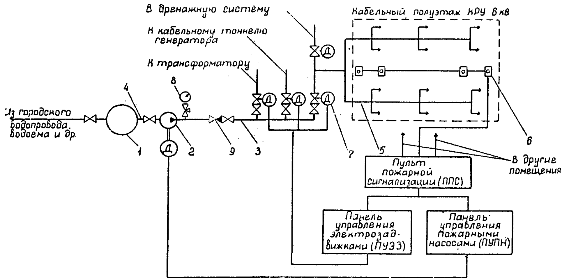
Принципиальная схема установки водяного пожаротушения:
